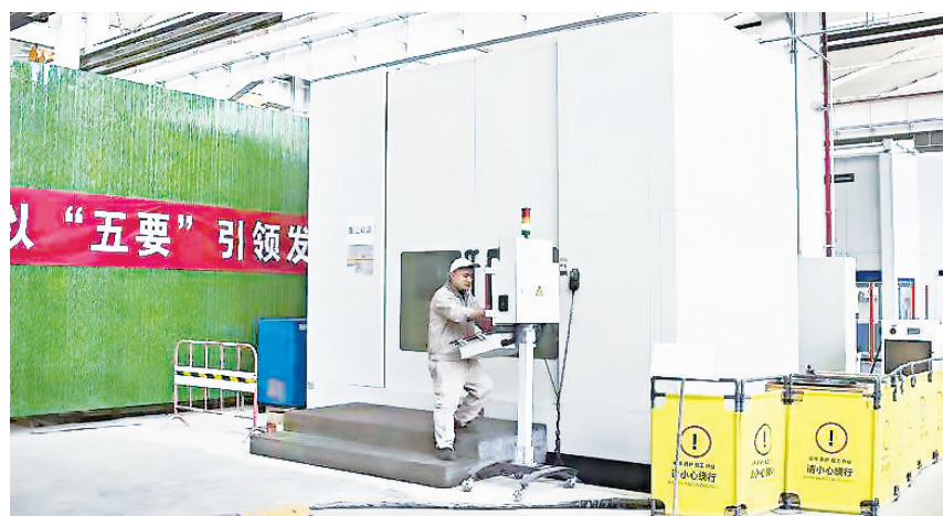
齿传分公司升级改造项目正按照集团公司“好、快、省”的要求全力推进,现场项目组争分夺秒,全力以赴确保项目按节点开展。目前,增速器车间设备基础制作完成36个,搬迁设备陆续进入调试阶段。上图为已安装完成的搬迁设备立式磨床。(齿传宣)
